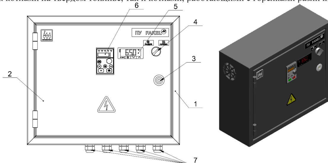
Рис. 2 Панель управления котлами FAKEL-M
