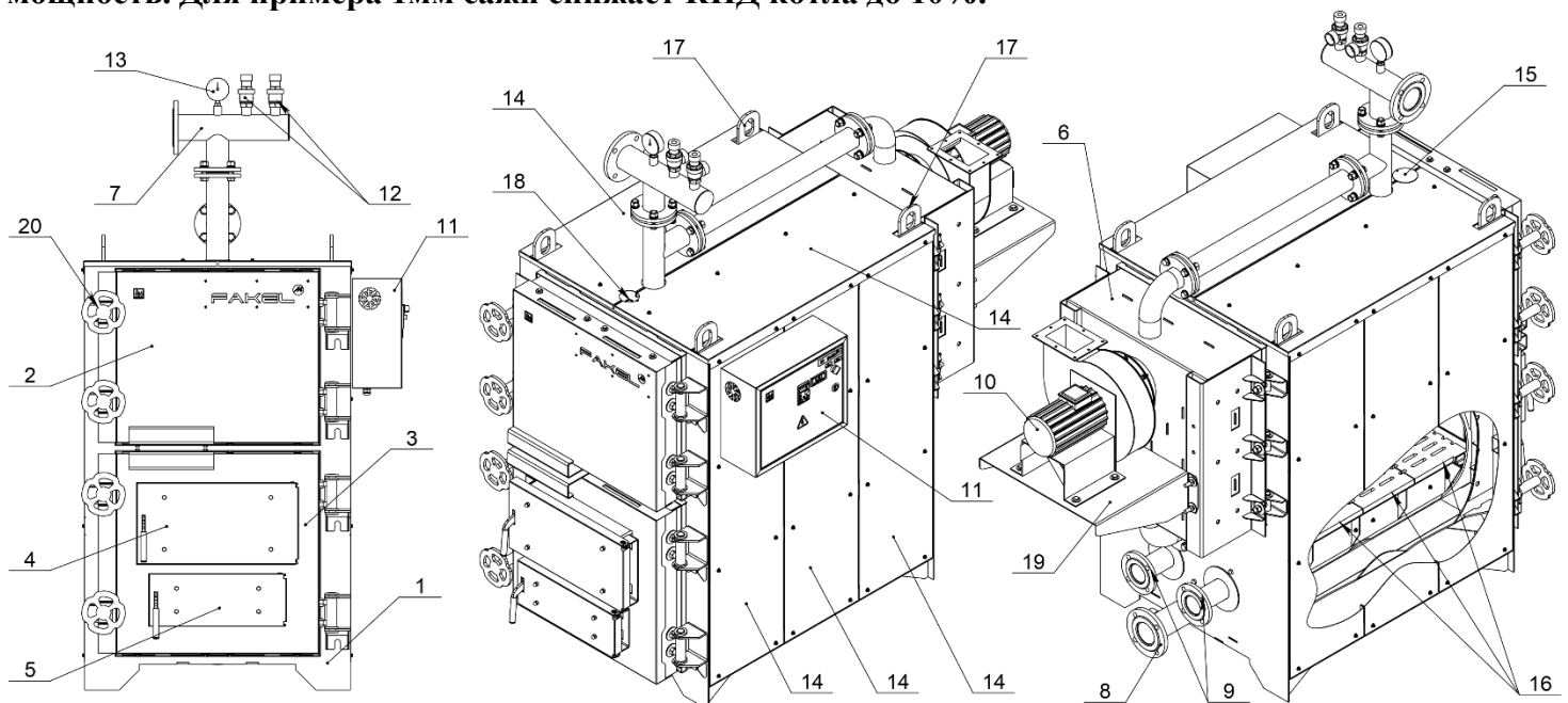
Рис. 1 Устройство котла FAKEL-М
